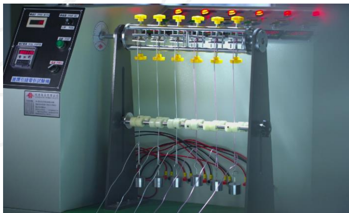
线材摇摆弯折测试
