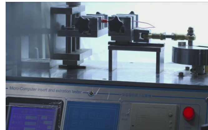
微电脑插头插拔测试
